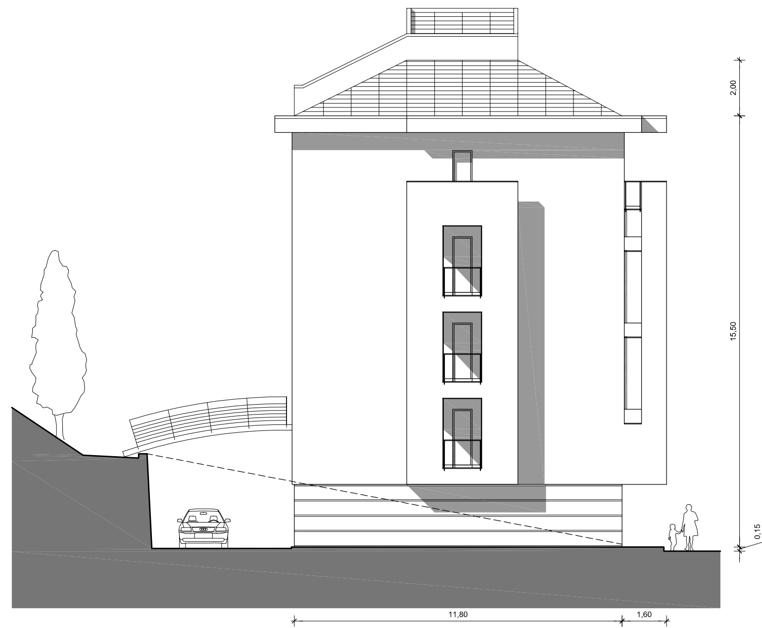
prospetto laterale
